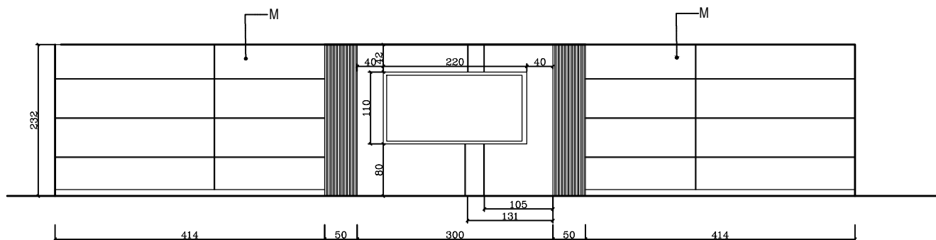
VIEW-D SC 1:20
