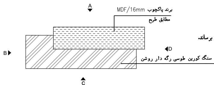
پلان کانتر پذیرایی
