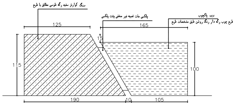
نمای کانتر پذیرش SC 1:10
