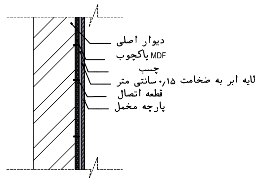
مقطع دیوار لمسه کوبی SC 1:5
